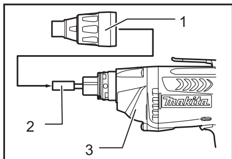
► 1. Anillo de bloqueo 2. Porta útil de entrada magnética 3. Caja del engranaje
