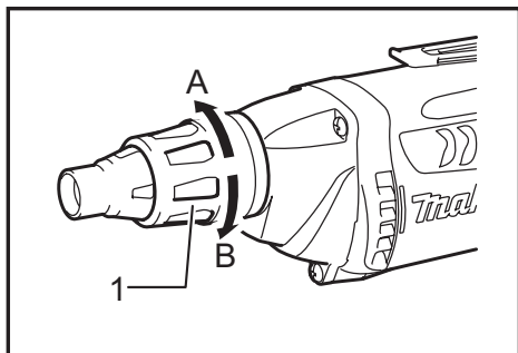
► 1. Locking ring
